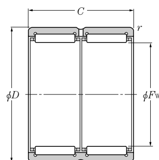
Type RNA69·R
