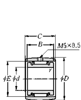
Type FRIS
