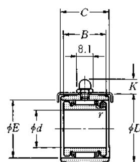
Type FRIS · SB (Non-separable)
