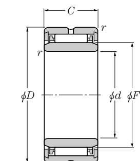
Type NA49 ( \phi d \leq 9\text{mm} )
