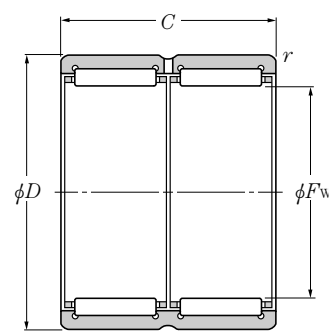
Type RNA69·R ( \phi F_w \geq 40\text{mm} )
