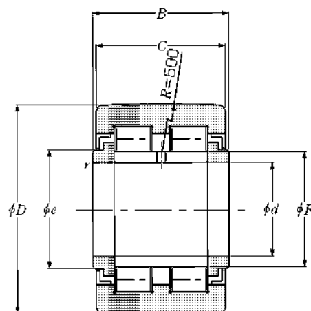
NUTW2 type
