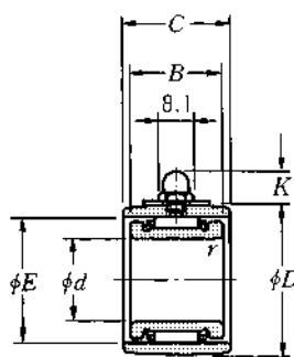
Type FRIS · SA (Separable)
